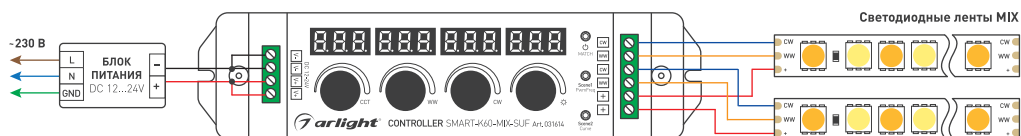
Рисунок 1. Схема подключения контроллера SMART-K60-MIX-SUF
